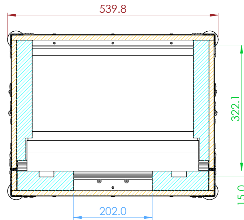
SECTION A-A SCALE 1 : 6
