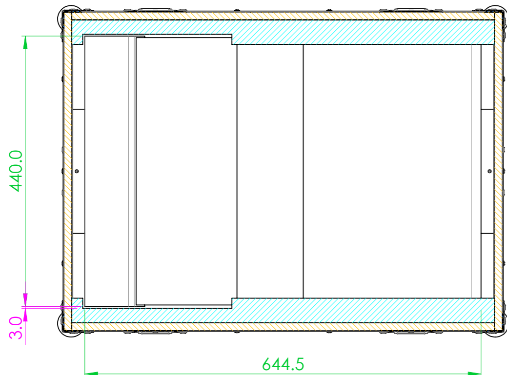
SECTION B-B SCALE 1 : 6
