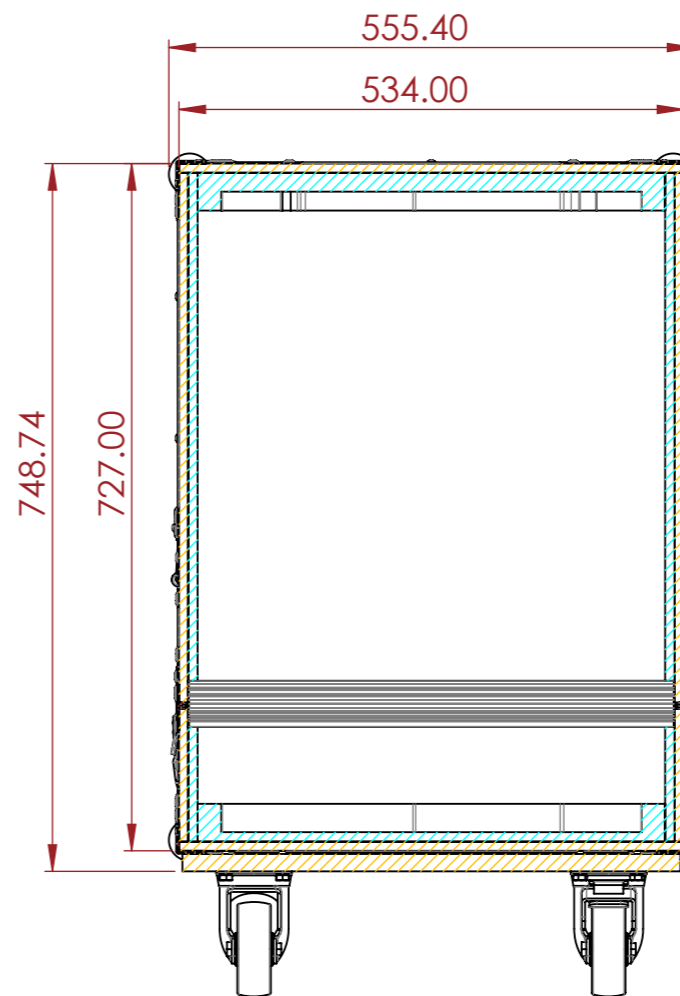
SECTION A-A
