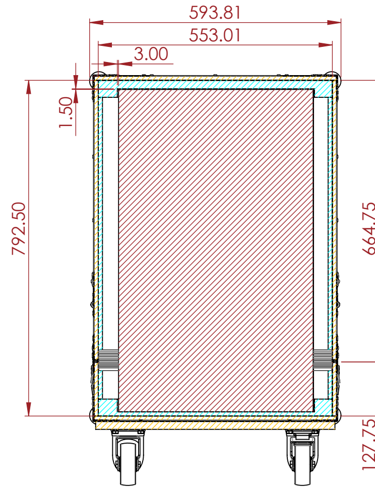
SECTION A-A SCALE 1 : 9
